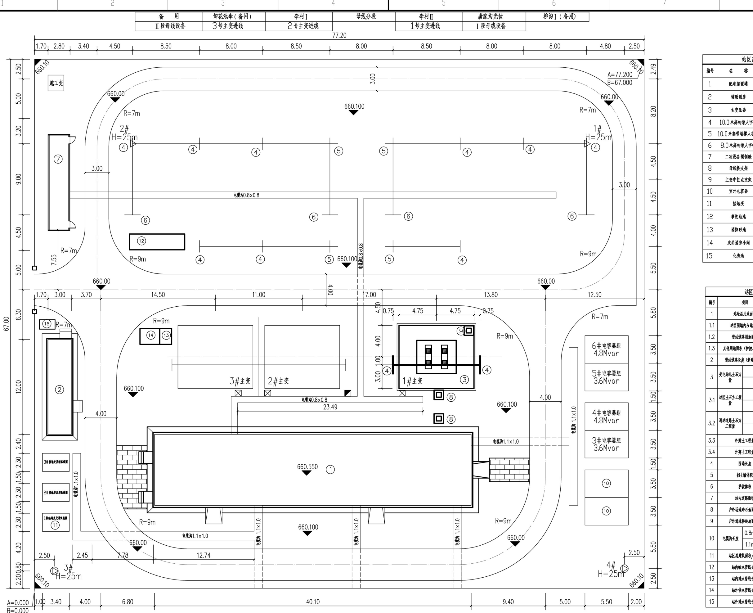
附图2：土建总平面及竖向布置图
